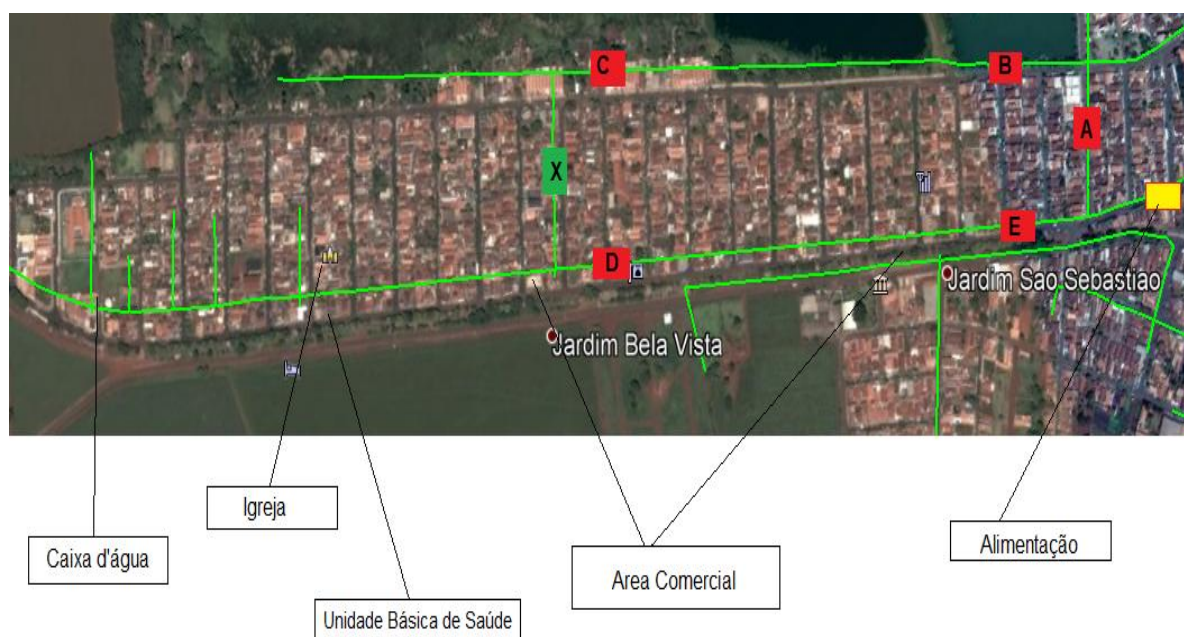
Figura 1: Configuração original da rede primária de alimentação de energia.
