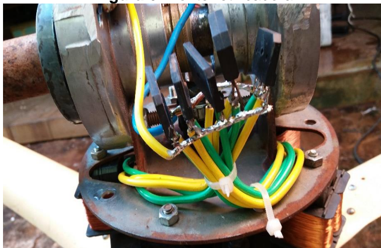
Figura 6: Ponte retificadora
