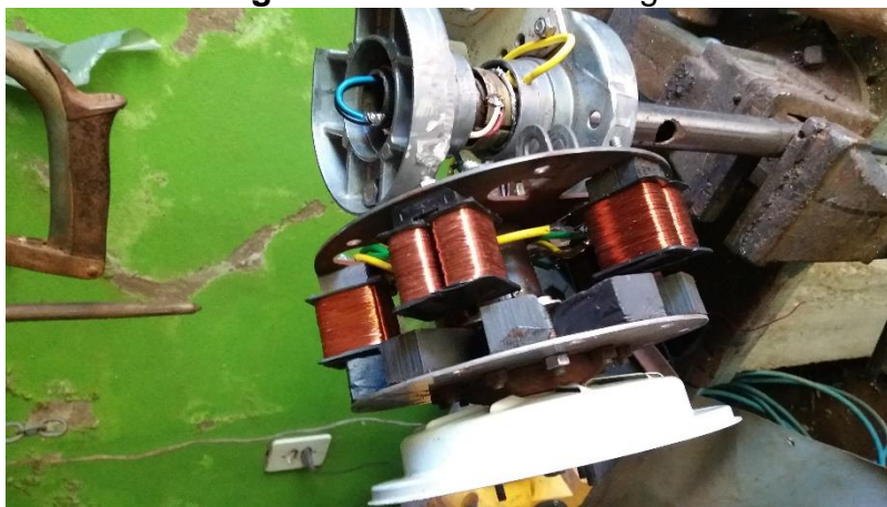
Figura 9: Gerador de energia
