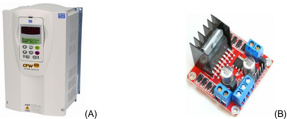
Figura 10: Inversores de frequência CFW 09 Weg (A), circuito eletrônico ponte H (B).
