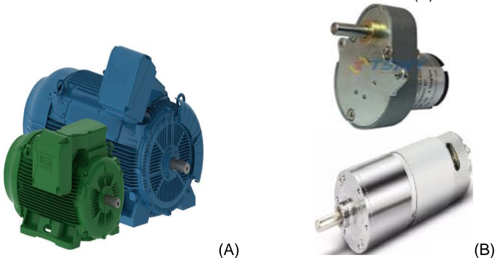
Figura 9: Motores de corrente alternada de 125CV 1100 RPM (A) e motores corrente contínua de 0.033 CV 80 RPM (B).
