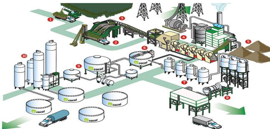
Figura1. Fluxograma da produção industrial no setor sucroalcooleiro
